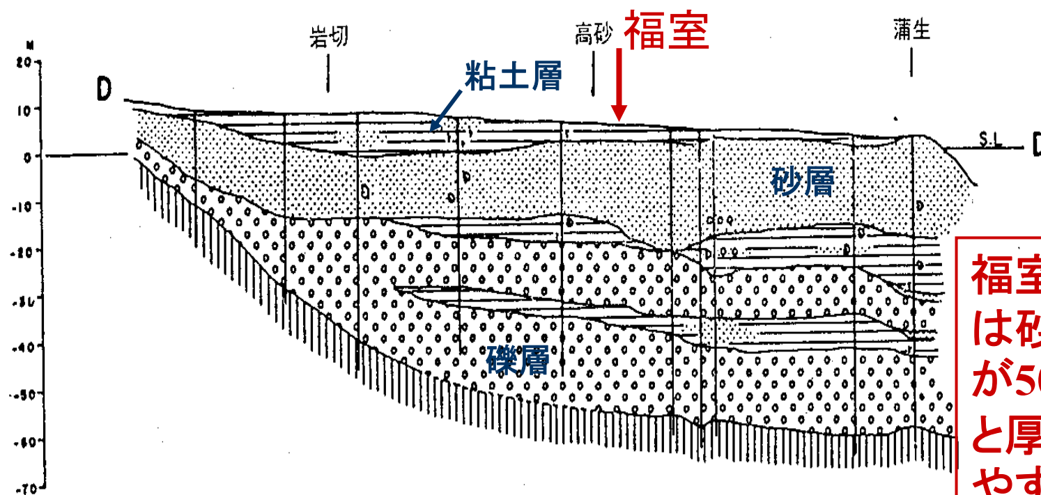
七北田川沿いの地質断面(地質調査所、S61年による)
