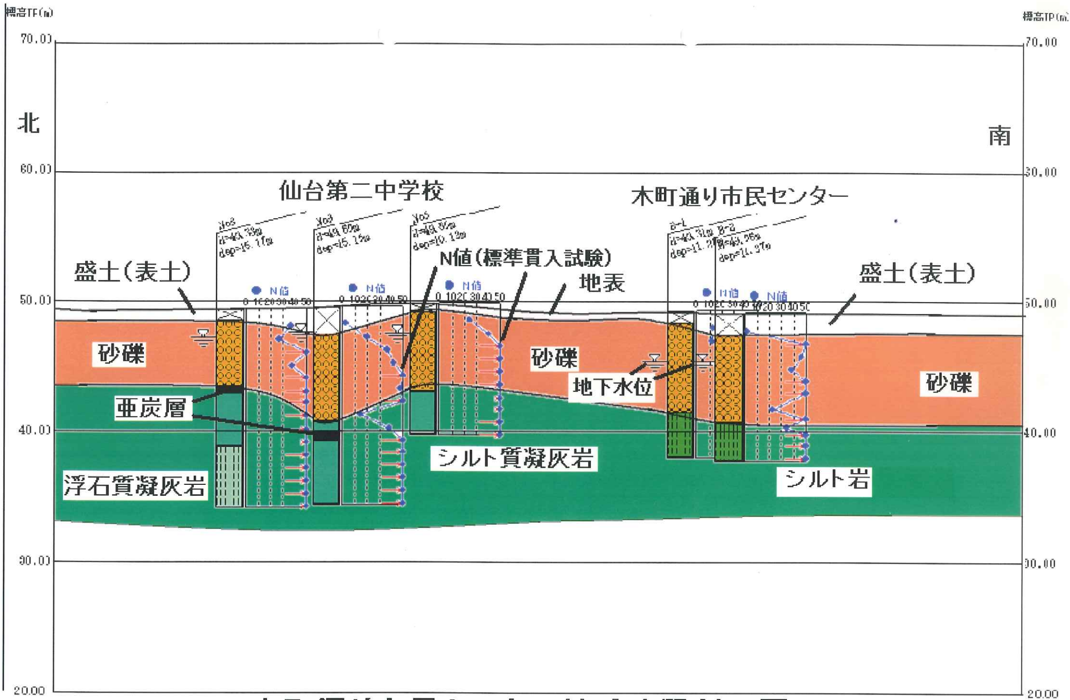
木町通り市民センター付近地質断面図
