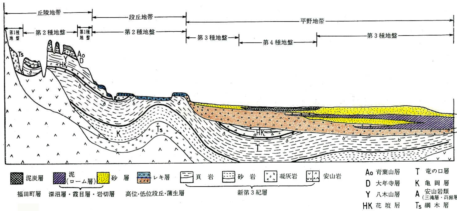
第III—2図 丘陵・段丘・平野間の表層地質・地盤種別を示す断面図
